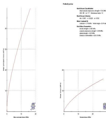
Slika 3. Određivanje parametara stenskog masiva za podinski pešćar Figure 3 Determination of rock mass parameters of the footwall sandstone
